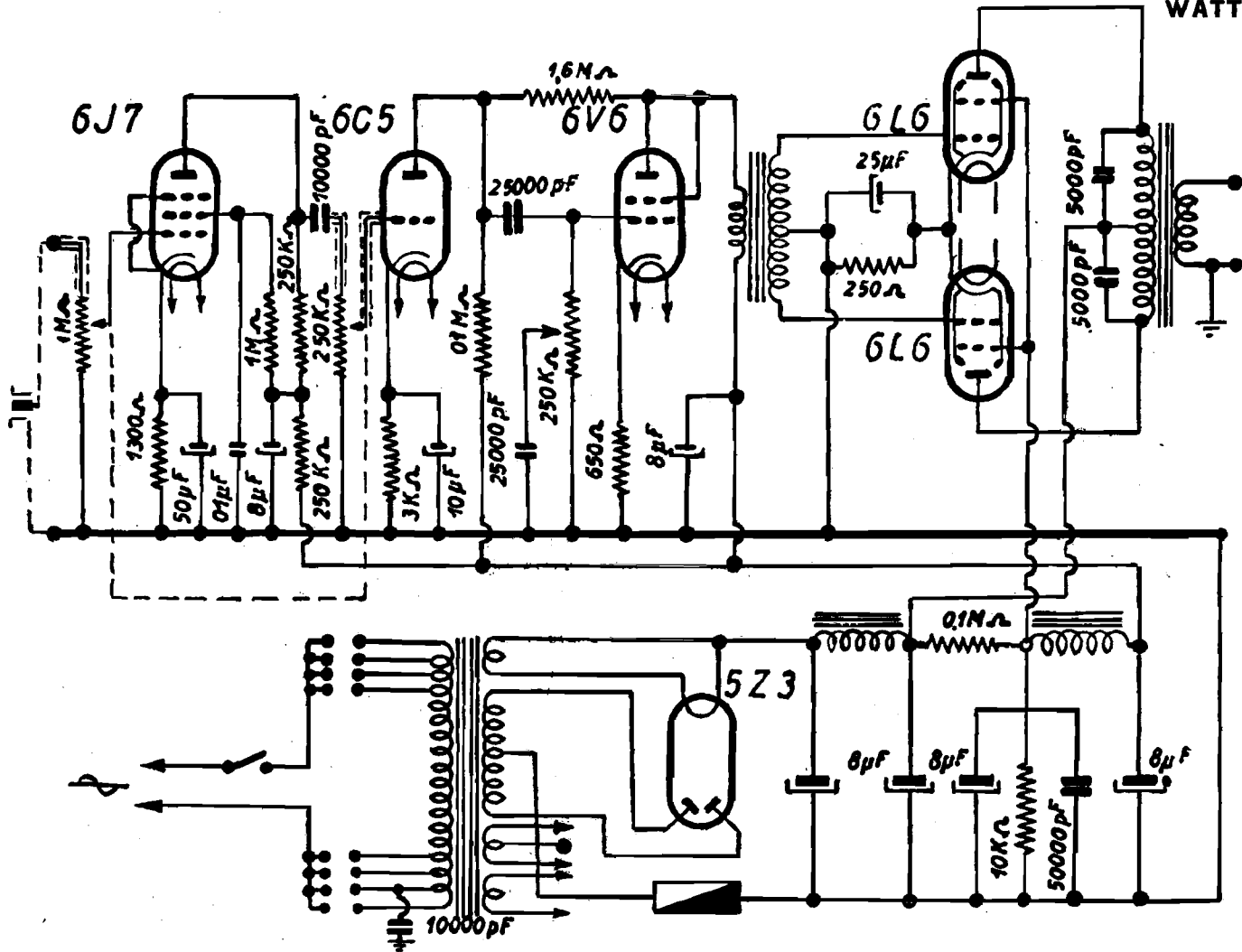
WATT RADIO - Amplificatore mod. W 630. Potenza 30 watt. Due 6L6 finali in classe AB2, funzionanti con 360 V di placca.
